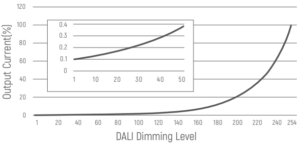
DALI 曲线
