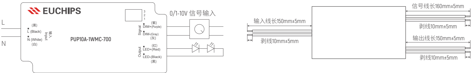
应用接线图
